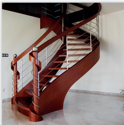
Schody Prudlik, Model: SP023. Ażurowe schody jednozabiegowe na policzkach giętych. Balustrada: stal nierdzewna z drewnianym pochwytem. Drewno: dąb bejcowany. Projekt i wykonanie: Schody Prudlik.
